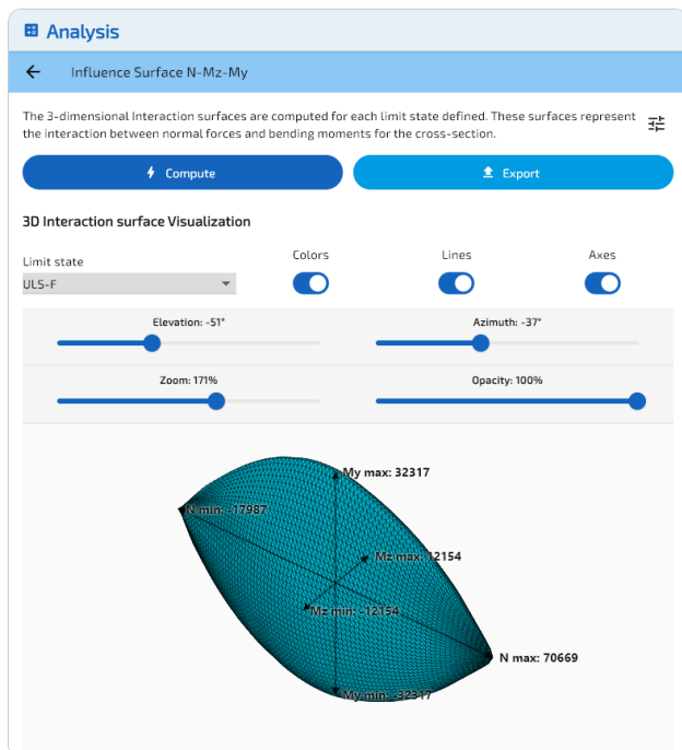
Figura 2: Superficie de interacao no ELU, triangulos coloridos.
