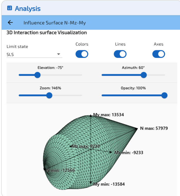
Figura 9: Superfície de interação no ELS, triângulos coloridos. Figura 10: Superfície de interação no ELS, vista em arame.
