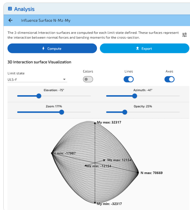
Figura 3: Superficie de interacao no ELU, vista em arame.
