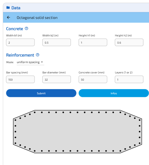
Figura 1: Secao octogonal: geometria e disposicao das armaduras.
