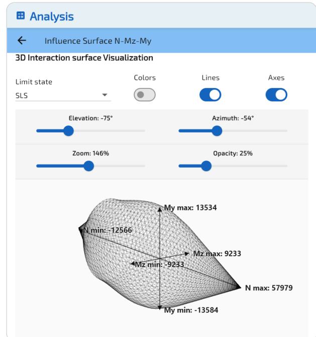
Figura 9: Superfície de interação no ELS, triângulos coloridos. Figura 10: Superfície de interação no ELS, vista em arame.
