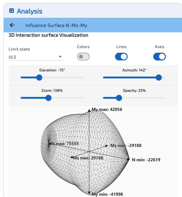
Figura 8: Superficie de interacao no ELU, vista em arame.
